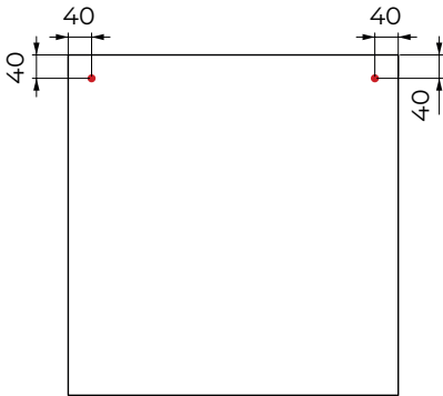
FOND 2 trous débouchants
