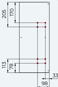
8 trous non débouchants pour les taquets
